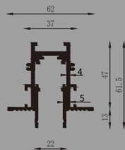
15款 预埋轨道型材图
