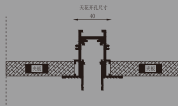
15款 预埋轨道型材固定
