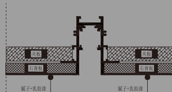
20-1款 预埋轨道型材完成
