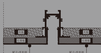
15款 预埋轨道型材完成
