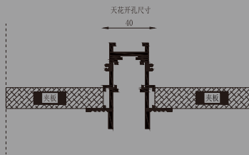
20-1款 预埋轨道型材固定
