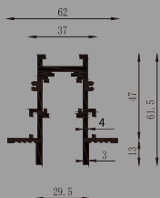
20-1款 预埋轨道型材图
