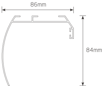
中罩壳尺寸
