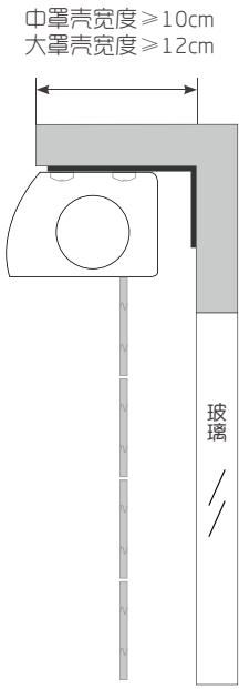
不带窗帘盒
