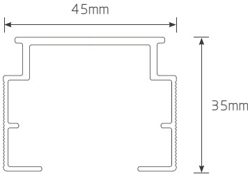
轨道截面尺寸
