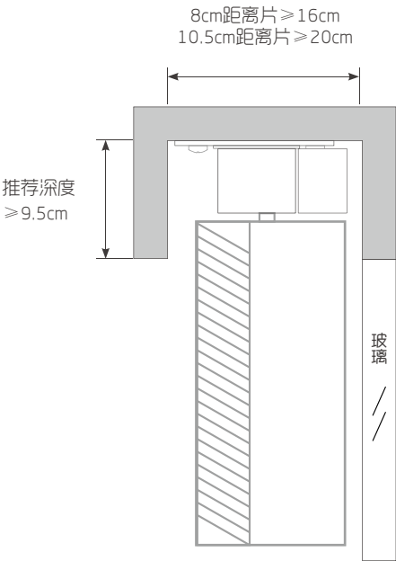
窗帘盒
