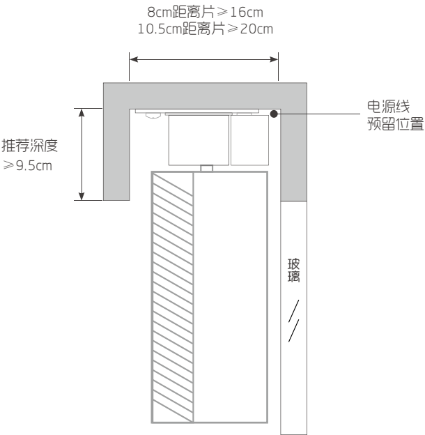
窗帘盒
