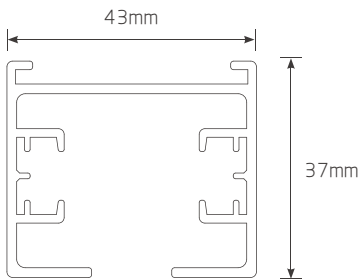
轨道截面尺寸
