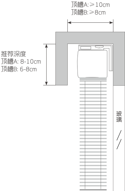
带窗帘盒
