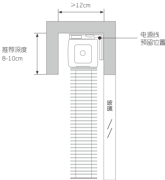
带窗帘盒
