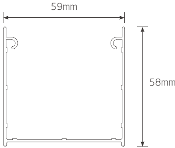
顶槽尺寸
