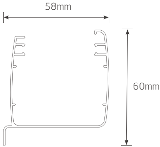
顶槽A尺寸
