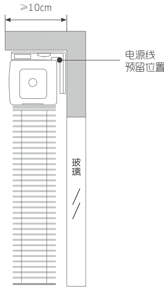
不带窗帘盒
