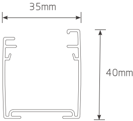
顶槽B尺寸
