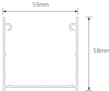
顶槽尺寸
