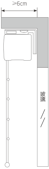
不带窗帘盒
