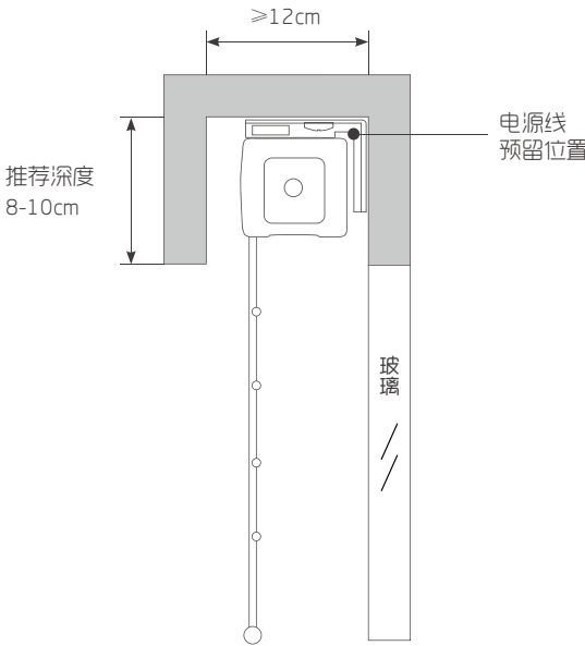
带窗帘盒
