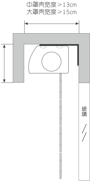
带窗帘盒
