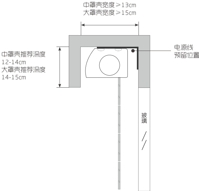
带窗帘盒
