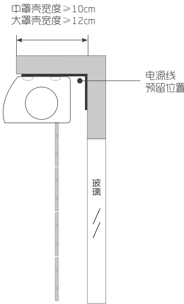
不带窗帘盒
