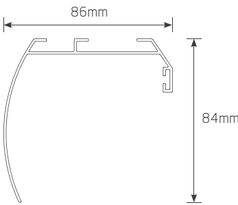
中罩壳尺寸
