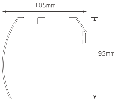
大罩壳尺寸
