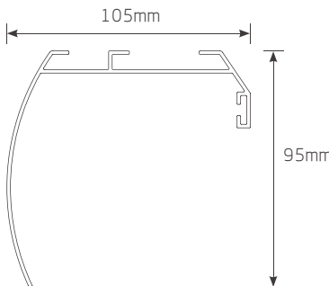
大罩壳尺寸
