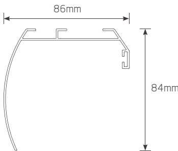
中罩壳尺寸
