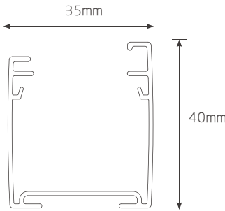
顶槽尺寸
