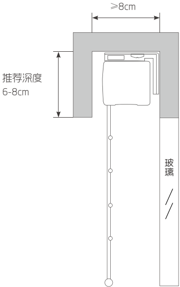
带窗帘盒
