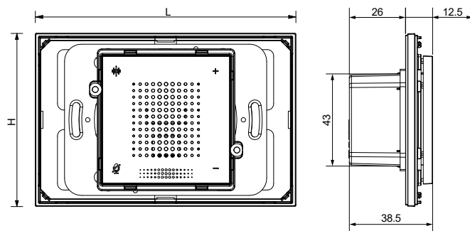
Montaggio con cornice: 122 x 77 (L x H) Montaggio senza cornice (*NF): 120 x 80 (L x H)
